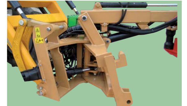
Movimiento lateral a derecha e izquierda tanto de la pinza vibradora como del paraguas interceptor. Adaptable a plantaciones de uno o varios pies de tronco.
